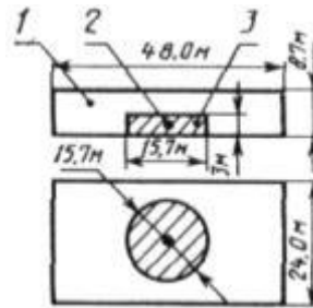
1 - помещение; 2 - аппарат; 3 - взрывоопасная зона
